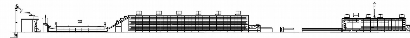
通心粉生产线MP-系列（麦粉、米或淀粉）； Macaroni pasta production line – MP Series
