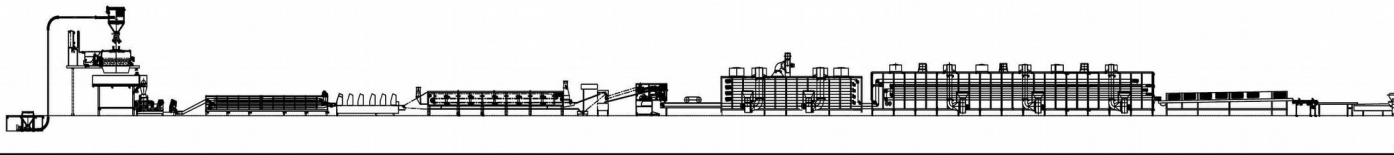
挂面生产线SN-系列 Stick noodle production line SN Series
