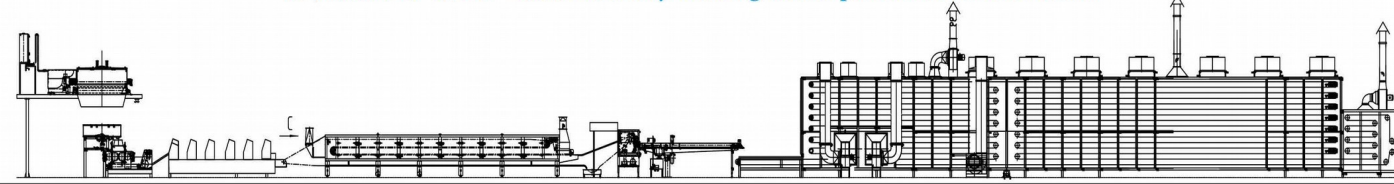
烘干方便面生产线DN-系列 Dried easy-cooking noodle production line DN-Series
