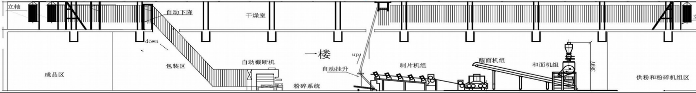
挂面生产线SN-系列 Stick noodle production line SN Series
